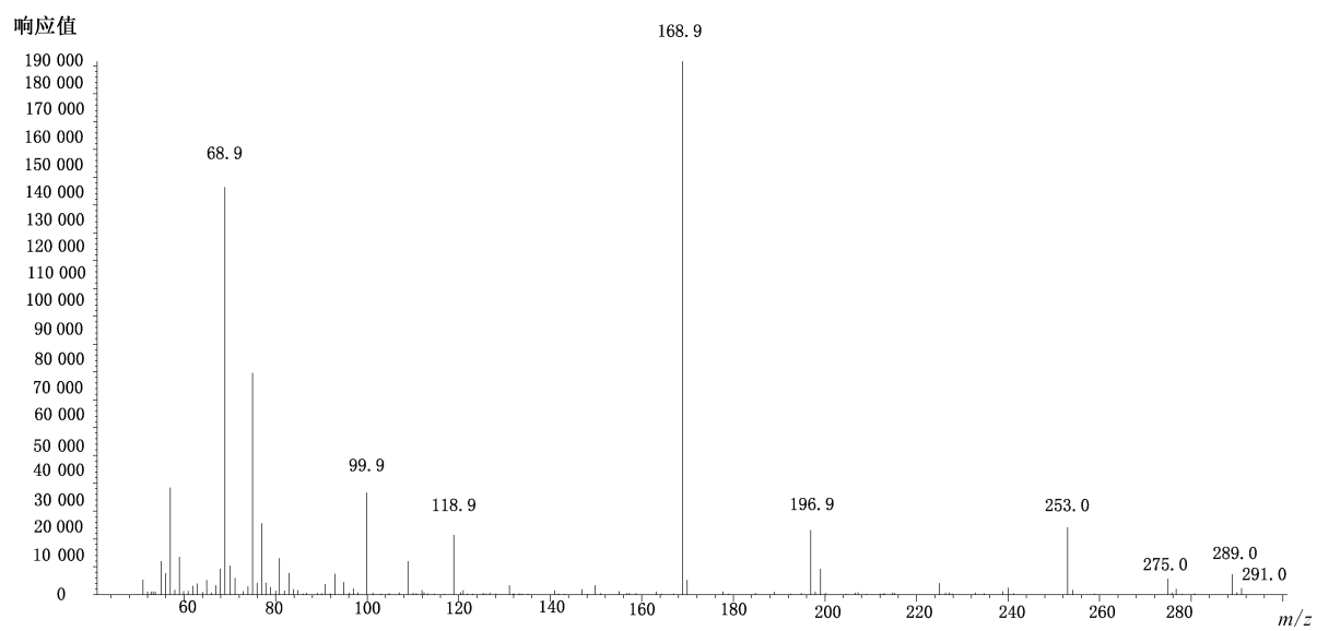
图 C.5 3-MCPD 衍生物质谱图 (200 \mu\text{g/L} )
