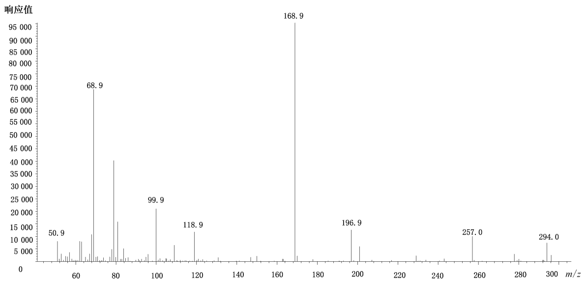
图 C.4 3-MCPD-D 5 衍生物质谱图(200 µg/L)
