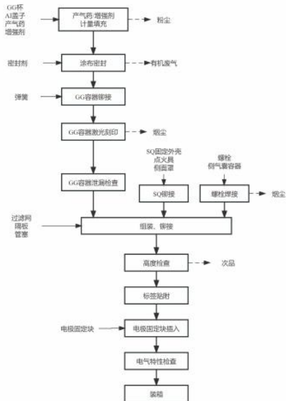
图 3-4 本项目 SIDE 线生产工艺及产污流程图
