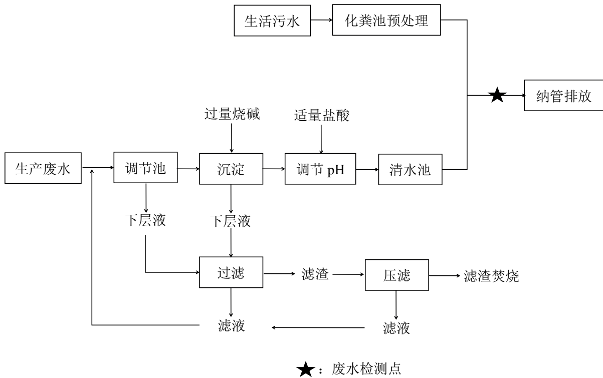
图 7-1-1 本项目废水处理工艺流程及废水监测点位示意图
