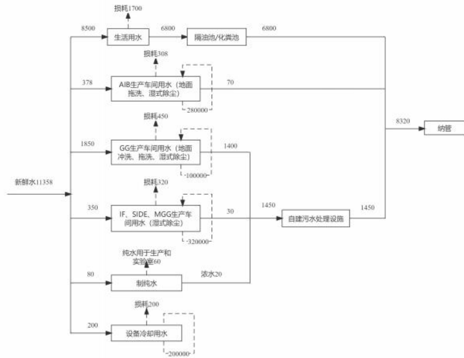
图 3-4 本项目水平衡图
