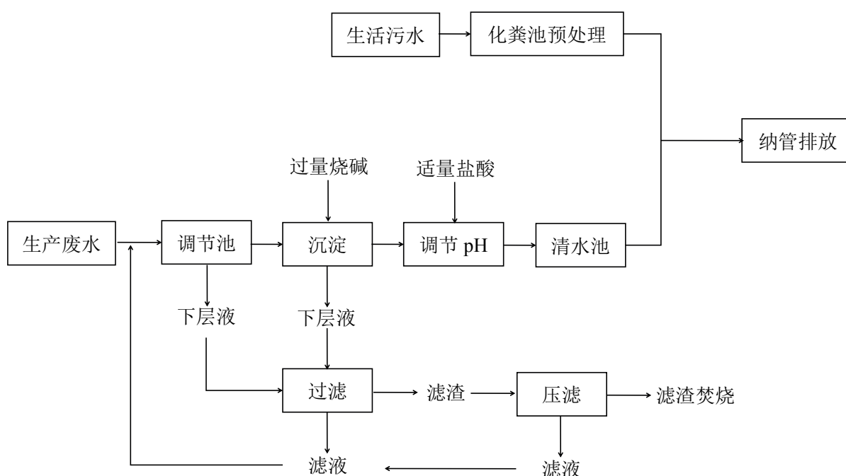
图 4-1 项目废水处理工艺流程图
