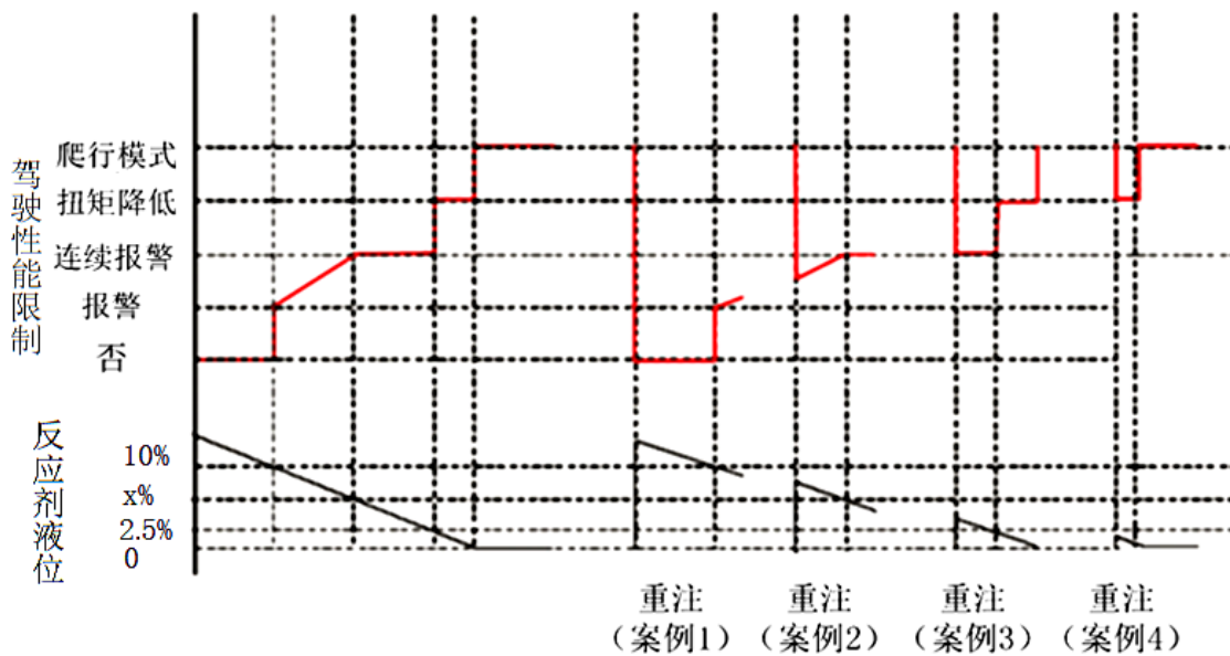
图 GB.2 监测到不同反应剂液位时，激活和解除激活的运行过程
